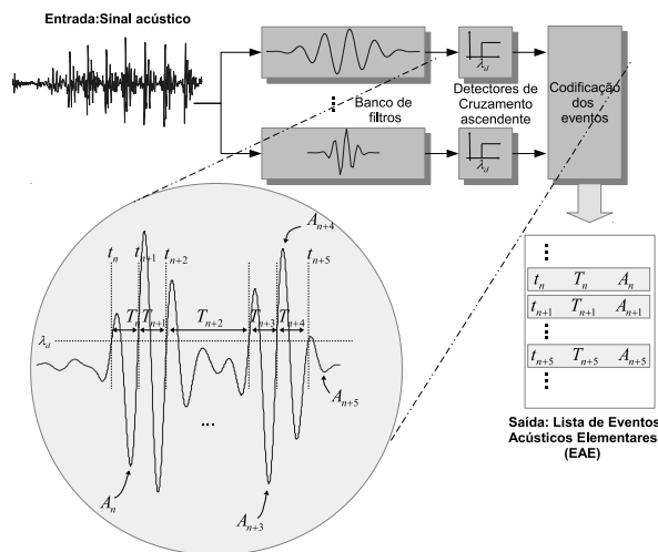
Figura 2: Ilustração do processamento para extração de Eventos Acústicos Elementares (EAE).
