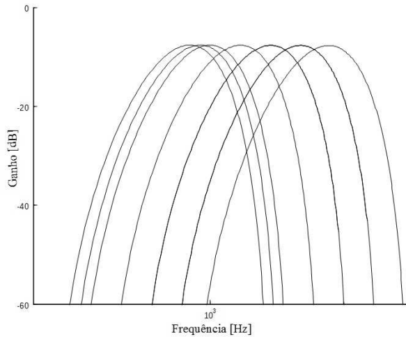
Figura 1: Resposta em frequência de sete dos vinte e oito filtros FIR implementados.
