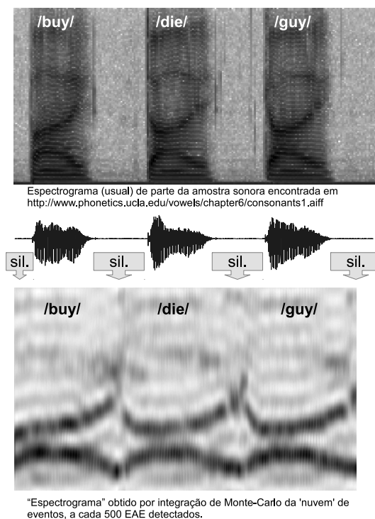
Figura 5: Ilustração do efeito de supressão dos intervalos de silêncio através da deformação não-linear da escala temporal - maior taxa de eventos acústicos detectados implica maior resolução temporal.
