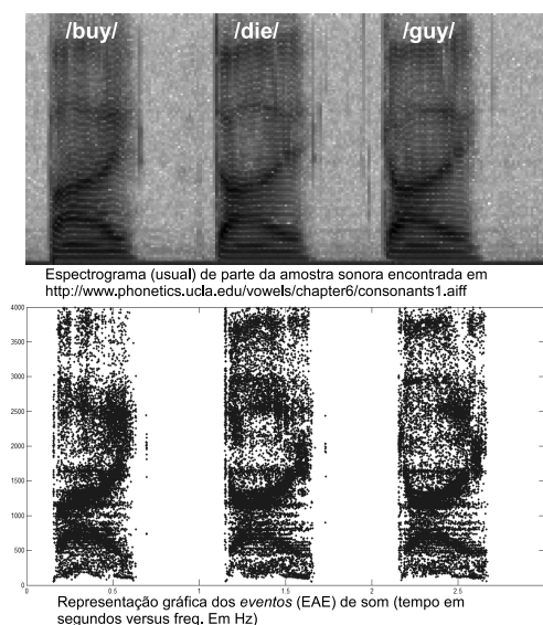
Figura 4: Comparação visual entre espectrograma convencional e o conjunto de EAE, representados por pontos no plano tempo \times frequência.
